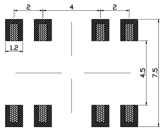
安装图 (PCB LAYOUT PLAN)
