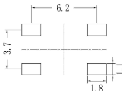
PCB印刷板 单位: mm
